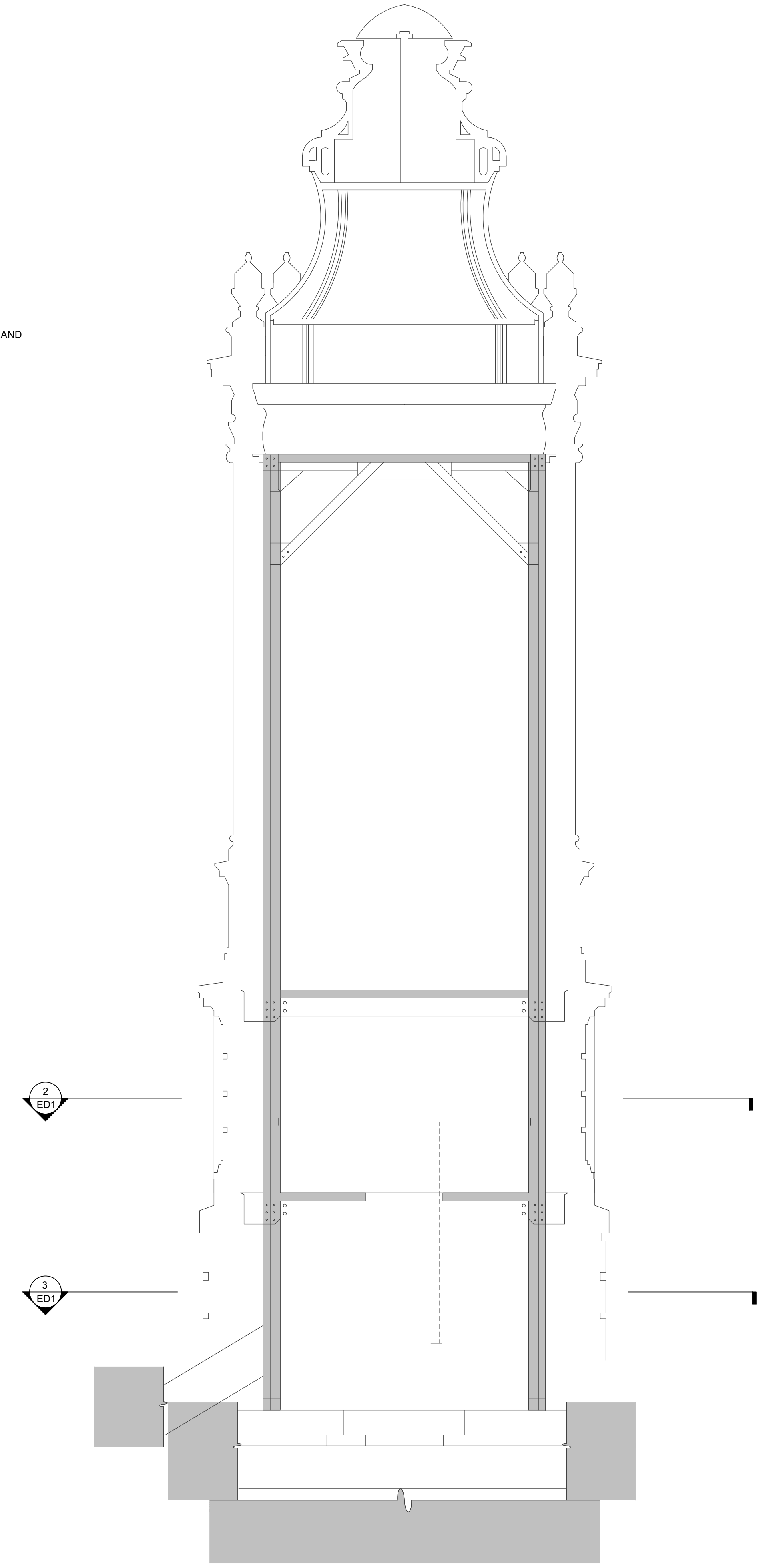
1 SECTION DETAIL ED1 SCALE: 1/2" = 1'-0"
