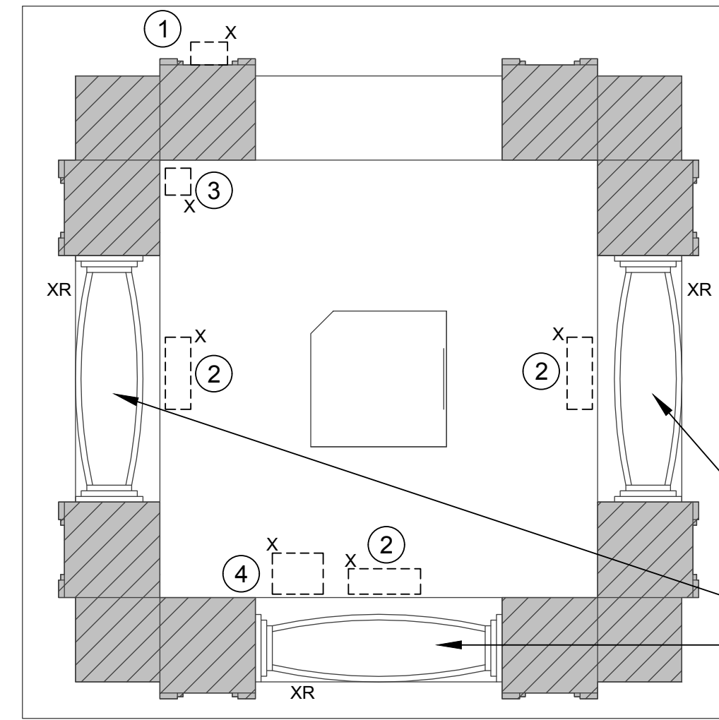
2 SECTION PLAN A ED1 SCALE: 1/2" = 1'-0"
