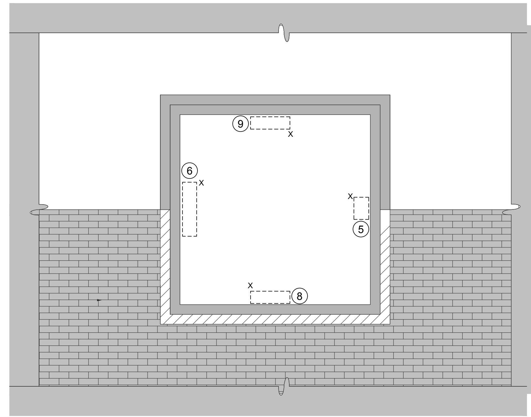
3 SECTION PLAN B ED1 SCALE: 1/2" = 1'-0"
